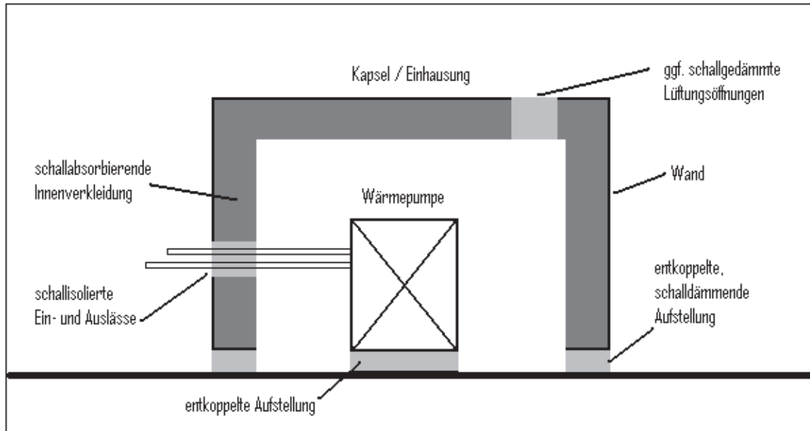
Abbildung 4: schematische Darstellung einer Kapselung
